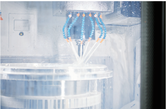
工具の全周から切削液をかけ、切削加工している様子
